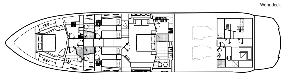
Wohndeck
